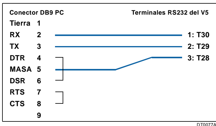
Figura 2.2: Cableado RS232.
